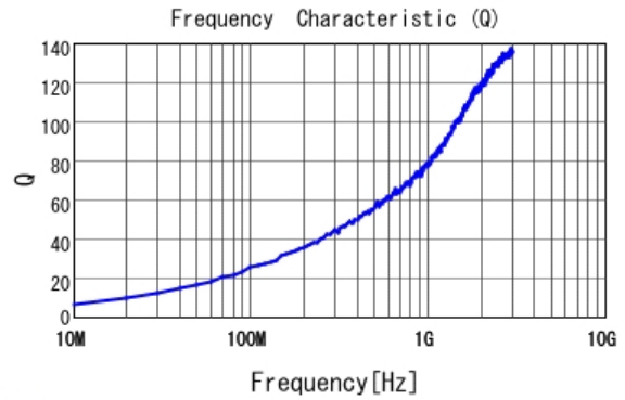
■ LQW15AN2N2C10 Q
