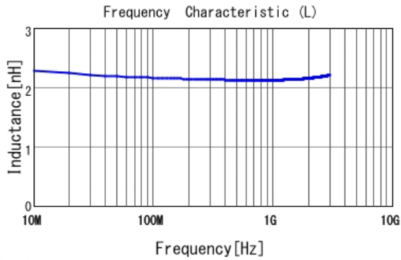
■ LQW15AN2N2C10 L
