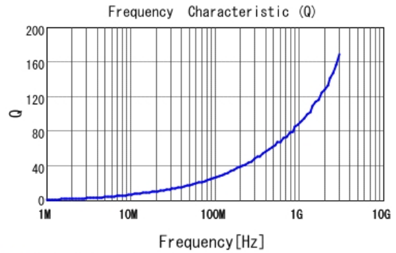
■ LQW15AN2N2G80 Q
