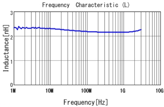
■ LQW15AN2N2G80 L
