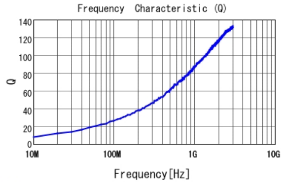
■ LQW15AN2N3C10 Q
