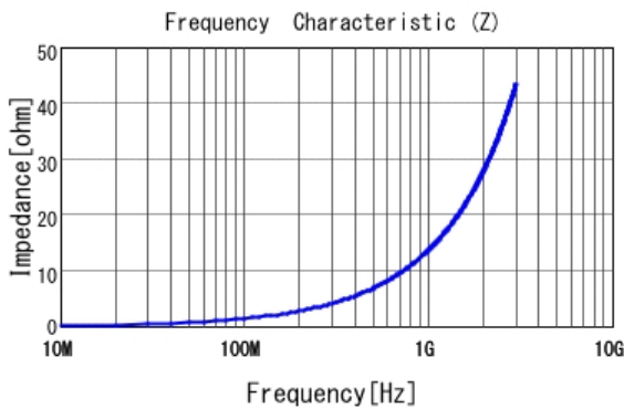
■ LQW15AN2N3C10 |Z|
