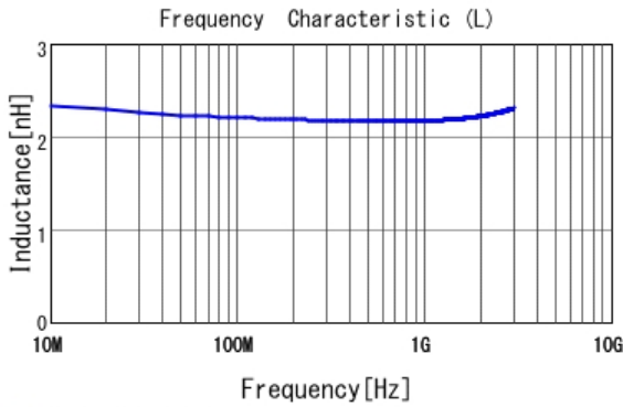
■ LQW15AN2N3C10 L
