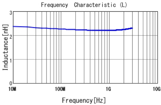
■ LQW15AN2N4B00 L
