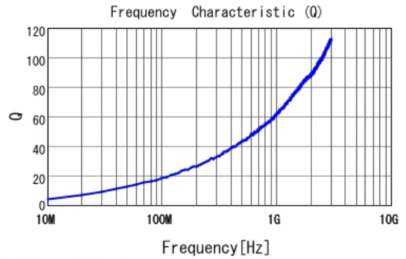
■ LQW15AN2N4B00 Q
