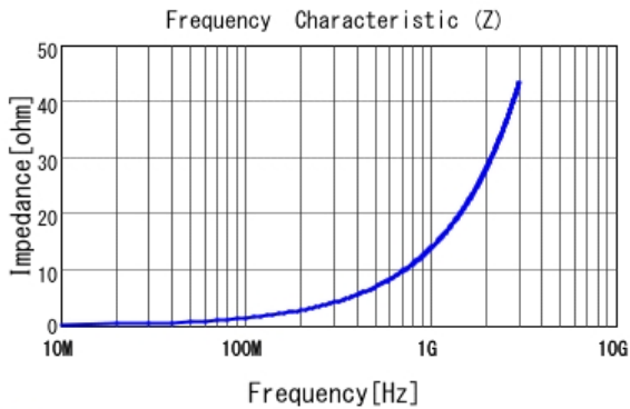
■ LQW15AN2N4B00 |Z|
