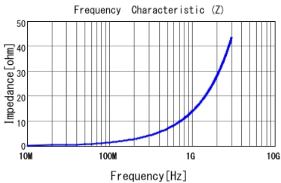
■ LQW15AN2N4C00 |Z|
