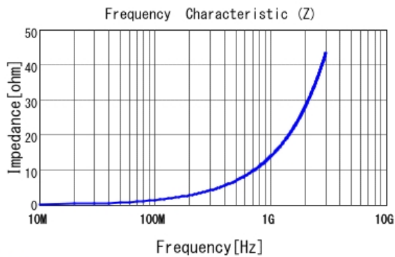
■ LQW15AN2N4D00 |Z|
