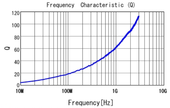
■ LQW15AN2N4D00 Q
