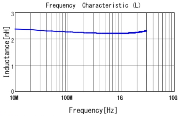
■ LQW15AN2N4D00 L
