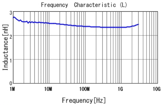
■ LQW15AN2N4G80 L
