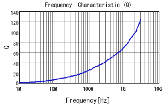
■ LQW15AN2N4G80 Q
