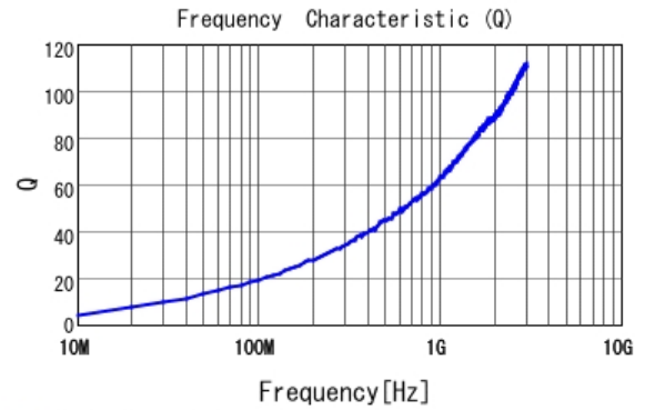
■ LQW15AN2N5B00 Q
