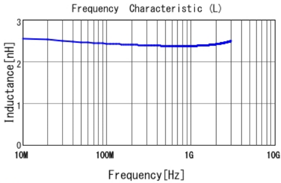
■ LQW15AN2N5B00 L
