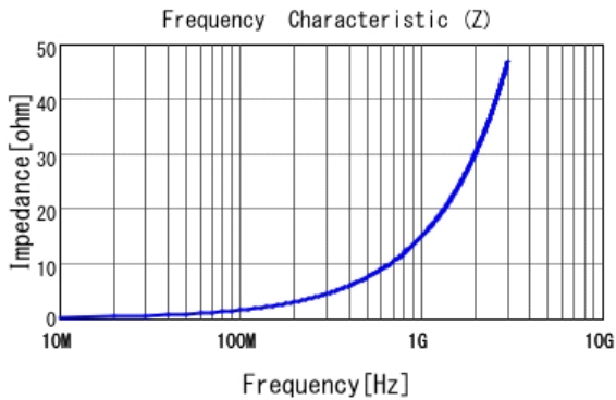
■ LQW15AN2N5B00 |Z|
