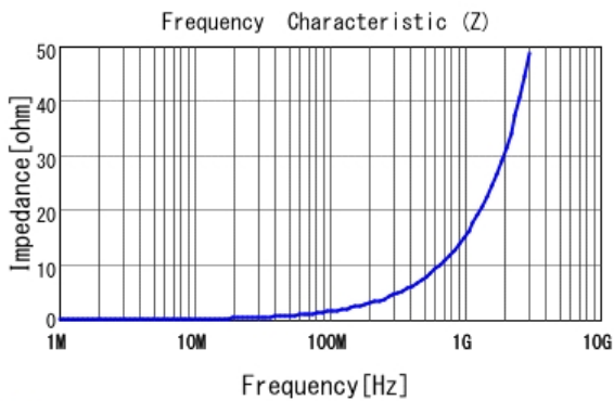
■ LQW15AN2N5G80 |Z|
