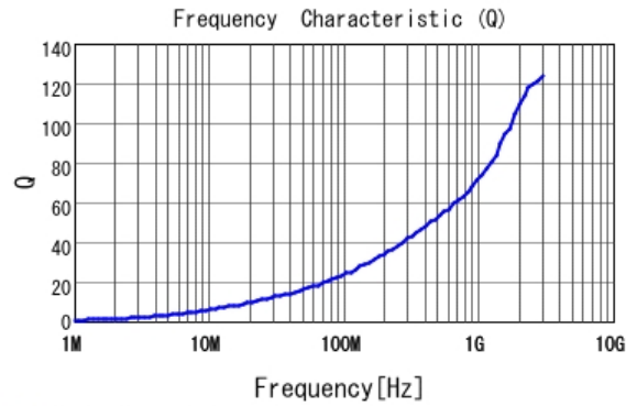
■ LQW15AN2N5G80 Q
