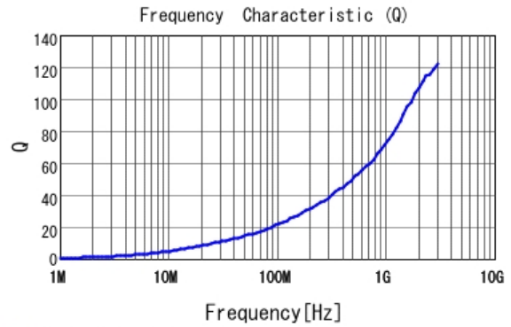
■ LQW15AN2N6G80 Q
