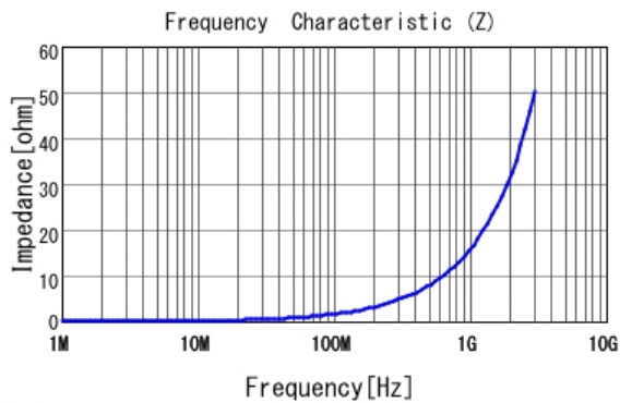
■ LQW15AN2N6G80 |Z|
