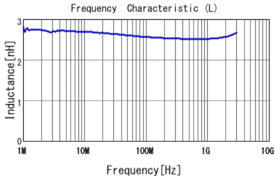
■ LQW15AN2N6G80 L
