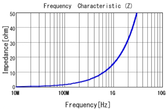
■ LQW15AN2N7B00 |Z|
