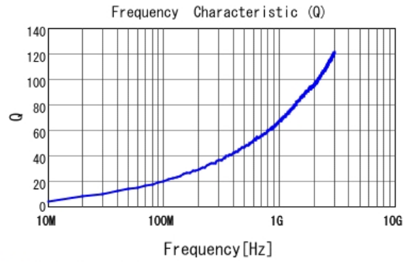
■ LQW15AN2N7B00 Q
