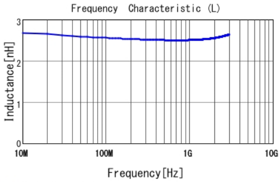
■ LQW15AN2N7B00 L
