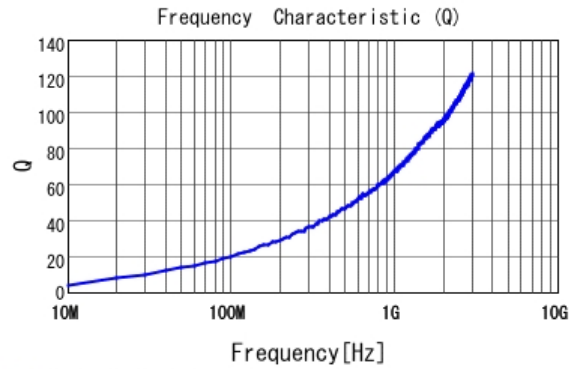
■ LQW15AN2N7C00 Q
