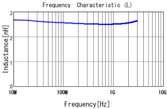
■ LQW15AN2N7C00 L
