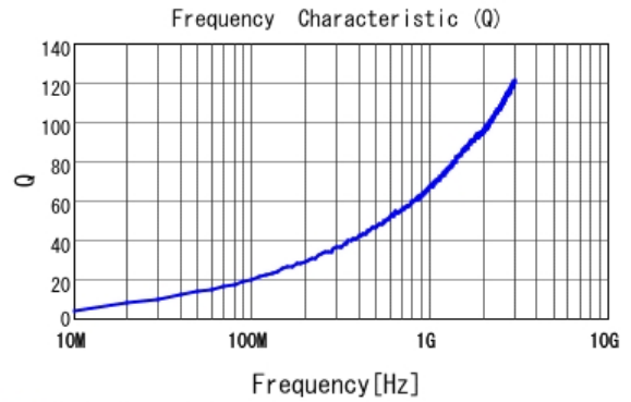
■ LQW15AN2N7D00 Q
