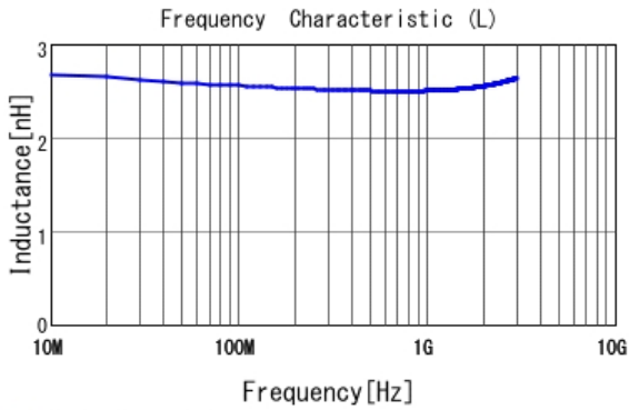
■ LQW15AN2N7D00 L
