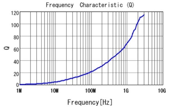
■ LQW15AN2N7G80 Q
