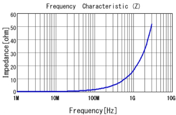
■ LQW15AN2N7G80 |Z|
