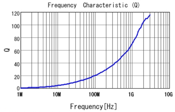
■ LQW15AN2N8G80 Q
