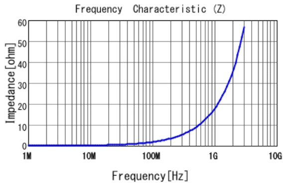
■ LQW15AN2N8G80 |Z|
