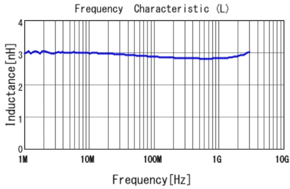
■ LQW15AN2N8G80 L
