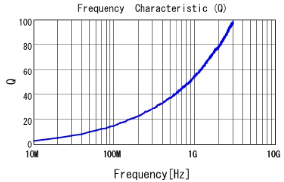
■ LQW15AN2N9C00 Q
