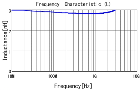
■ LQW15AN2N9C00 L
