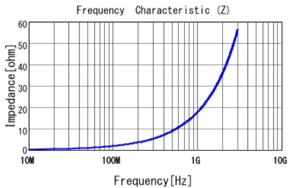
■ LQW15AN2N9C00 |Z|
