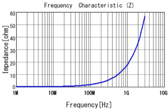
■ LQW15AN2N9G80 |Z|
