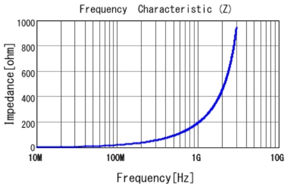
■ LQW15AN30NG00 |Z|
