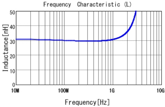
■ LQW15AN30NG00 L
