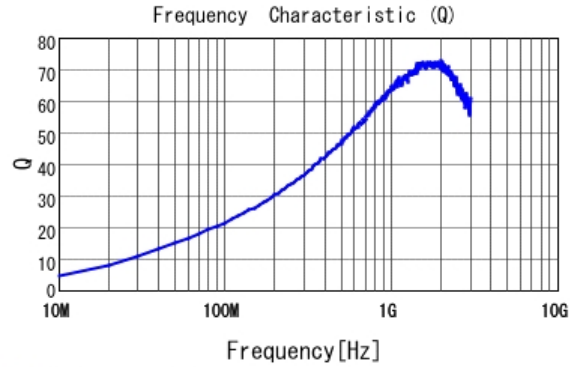
■ LQW15AN30NG00 Q
