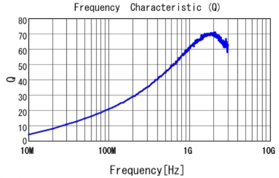
■ LQW15AN33NG00 Q
