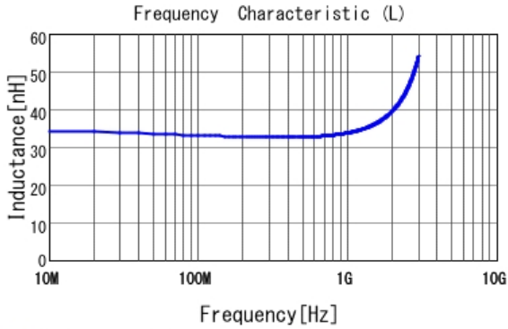
■ LQW15AN33NG00 L
