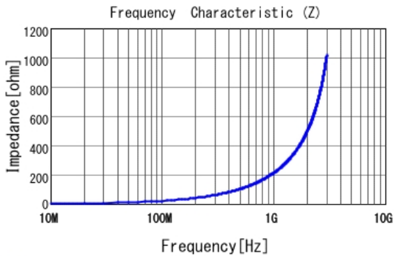
■ LQW15AN33NG00 |Z|
