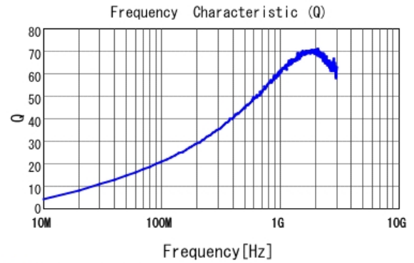
■ LQW15AN33NJ00 Q
