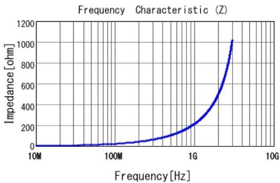
■ LQW15AN33NJ00 |Z|
