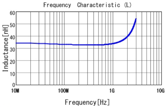
■ LQW15AN33NJ00 L
