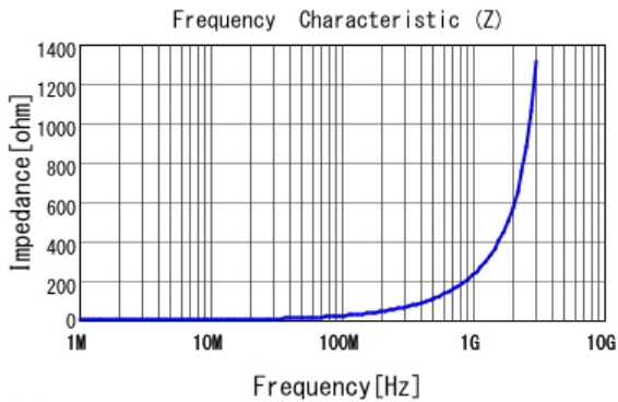
■ LQW15AN36NG80 |Z|
