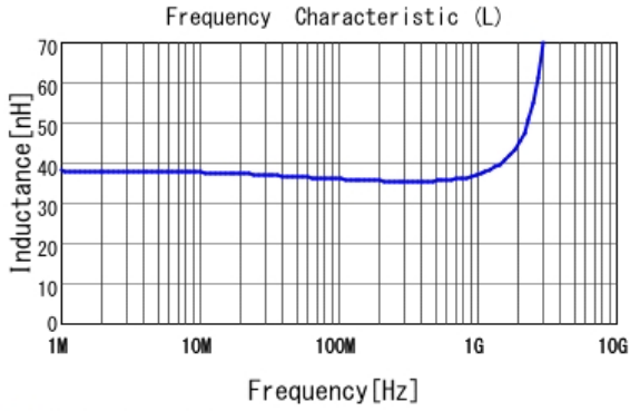
■ LQW15AN36NG80 L
