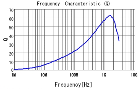
■ LQW15AN36NG80 Q
