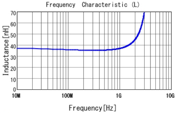
■ LQW15AN36NJ00 L
