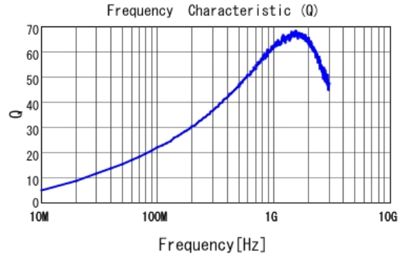
■ LQW15AN36NJ00 Q
