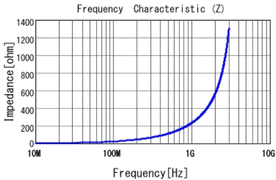
■ LQW15AN36NJ00 |Z|
