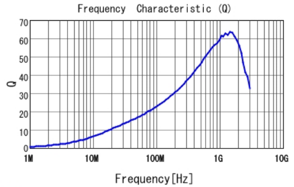
■ LQW15AN39NG80 Q
