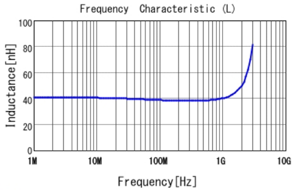
■ LQW15AN39NG80 L
