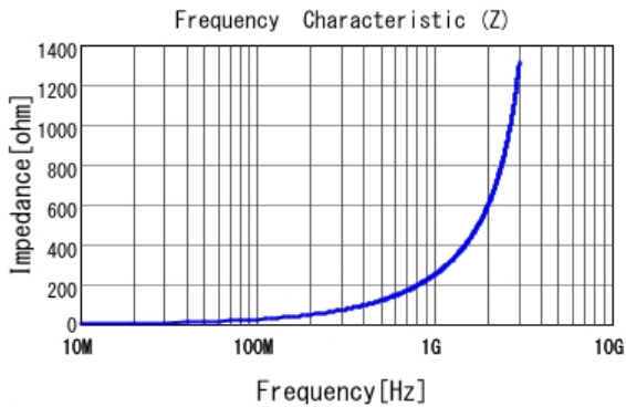
■ LQW15AN39NJ0Z |Z|
