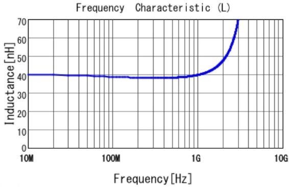
■ LQW15AN39NJ0Z L
