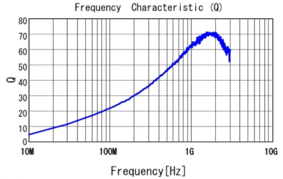
■ LQW15AN39NJ0Z Q
