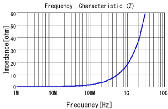
■ LQW15AN3N0G80 |Z|
