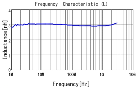
■ LQW15AN3N0G80 L
