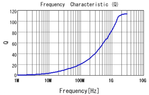
■ LQW15AN3N0G80 Q
