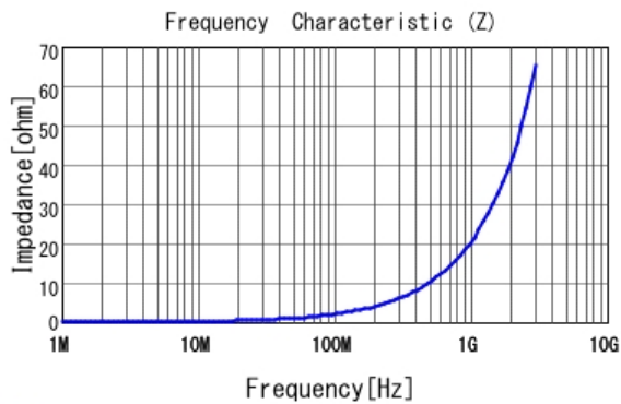
■ LQW15AN3N3B80 |Z|
