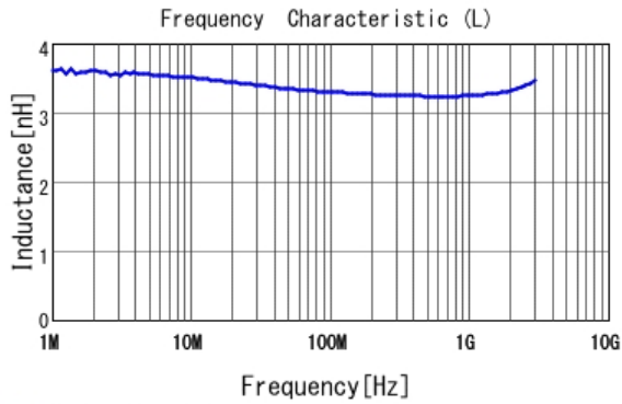
■ LQW15AN3N3B80 L
