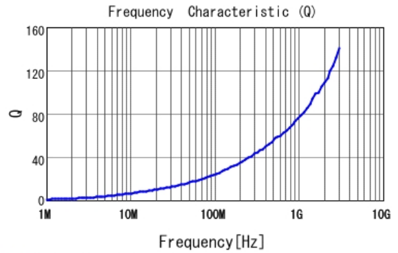
■ LQW15AN3N3B80 Q
