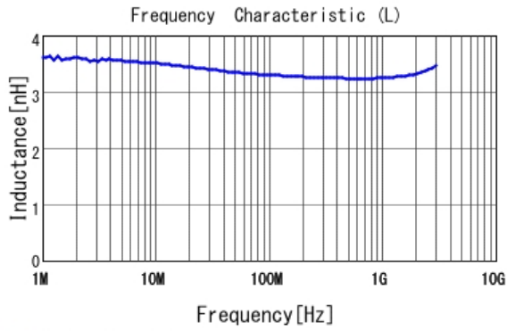
■ LQW15AN3N3G80 L
