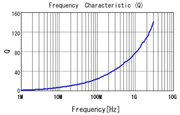
■ LQW15AN3N3G80 Q
