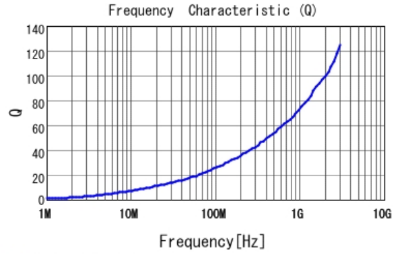
■ LQW15AN3N4B80 Q
