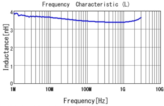
■ LQW15AN3N4B80 L
