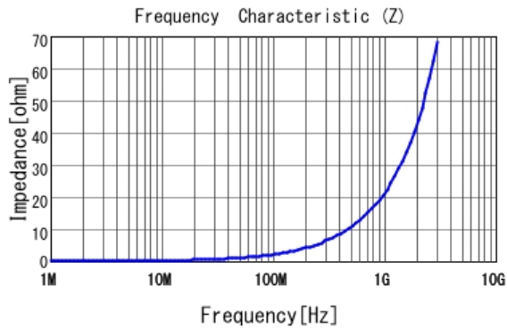
■ LQW15AN3N4B80 |Z|
