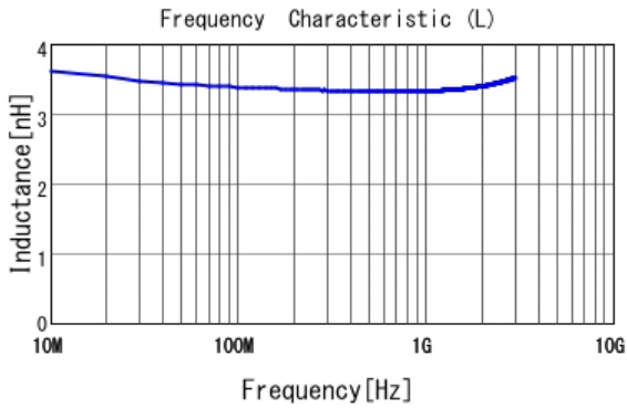
■ LQW15AN3N4C10 L
