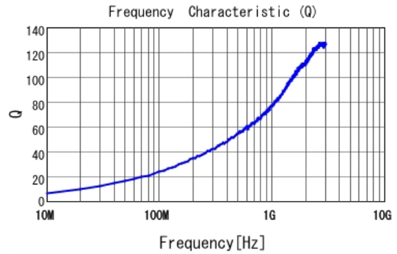
■ LQW15AN3N4C10 Q
