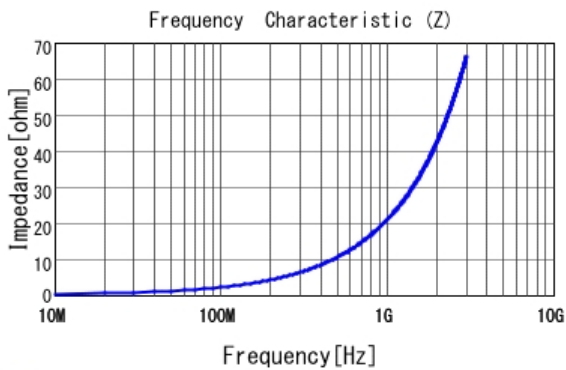
■ LQW15AN3N4C10 |Z|
