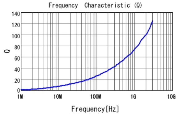
■ LQW15AN3N4G80 Q
