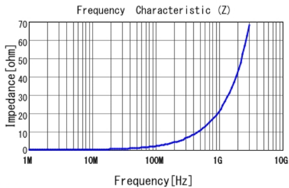
■ LQW15AN3N4G80 |Z|
