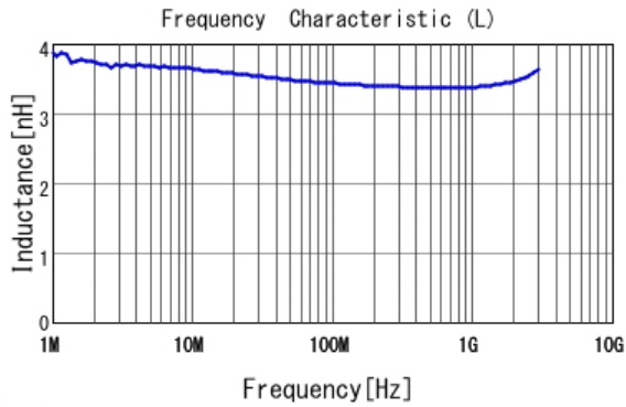
■ LQW15AN3N4G80 L
