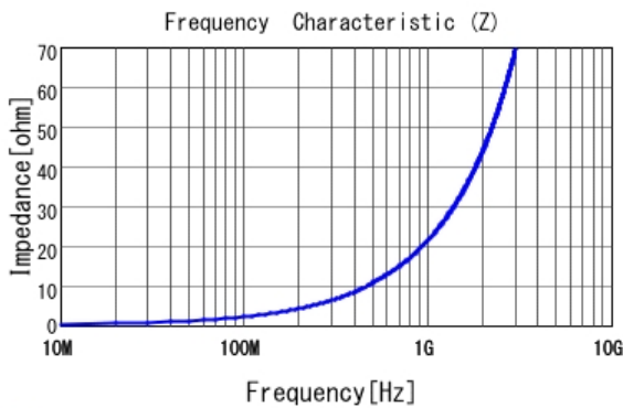
■ LQW15AN3N5C10 |Z|
