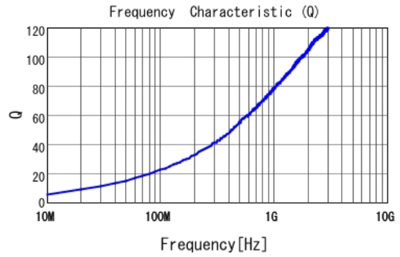
■ LQW15AN3N5C10 Q
