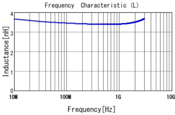
■ LQW15AN3N5C10 L
