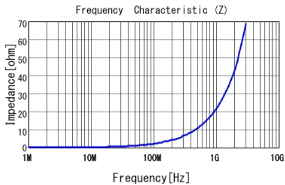
■ LQW15AN3N5G80 |Z|
