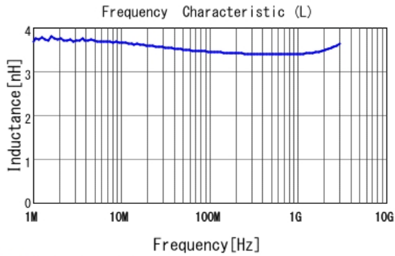
■ LQW15AN3N5G80 L
