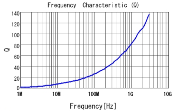
■ LQW15AN3N5G80 Q
