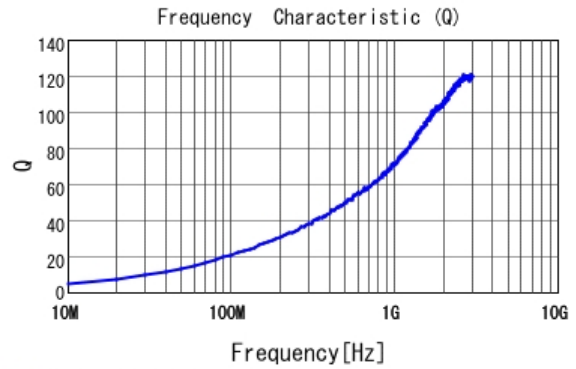
■ LQW15AN3N6C10 Q
