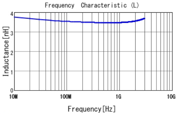
■ LQW15AN3N6C10 L
