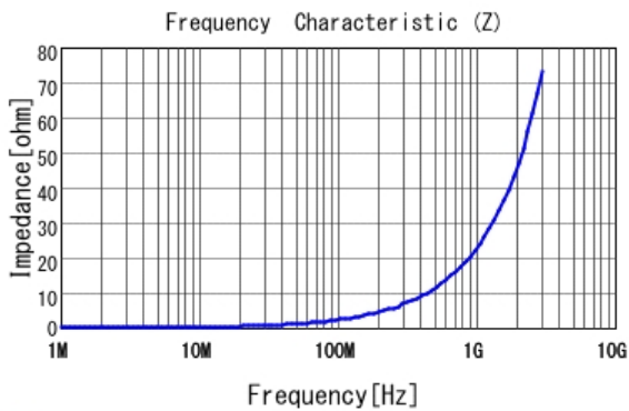
■ LQW15AN3N6G80 |Z|
