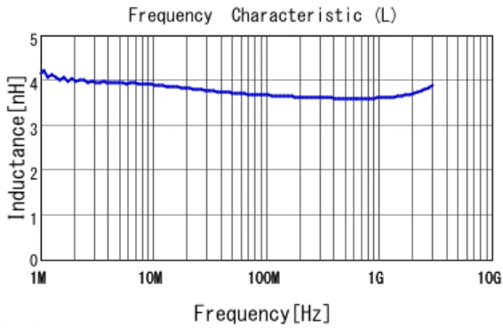
■ LQW15AN3N6G80 L
