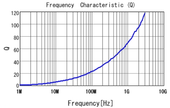
■ LQW15AN3N6G80 Q
