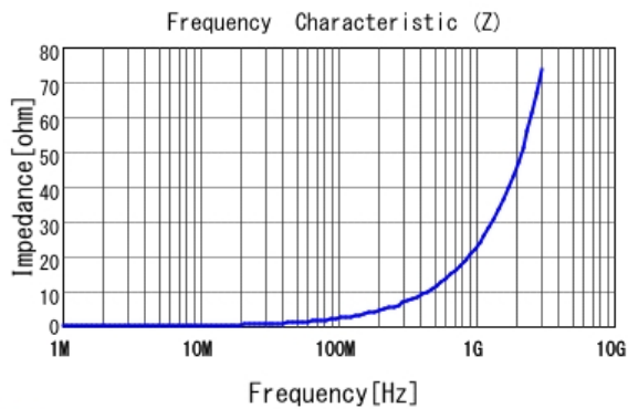
■ LQW15AN3N7G80 |Z|
