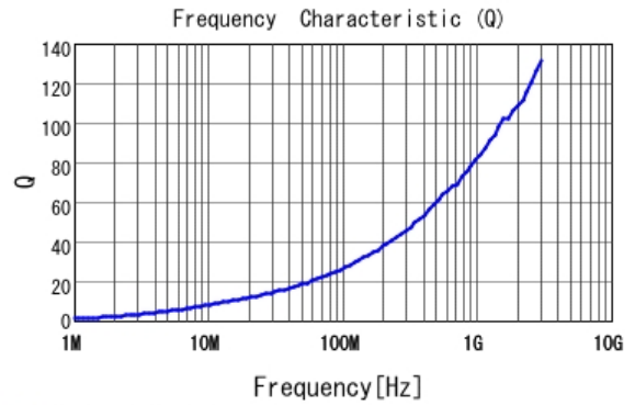
■ LQW15AN3N7G80 Q
