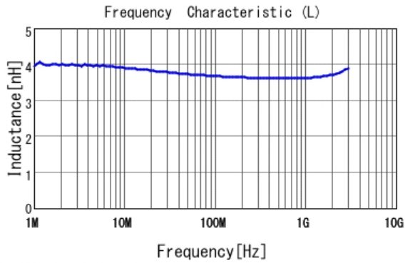
■ LQW15AN3N7G80 L
