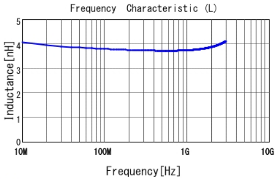
■ LQW15AN3N8C10 L
