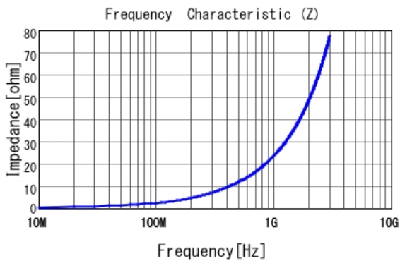
■ LQW15AN3N8C10 |Z|
