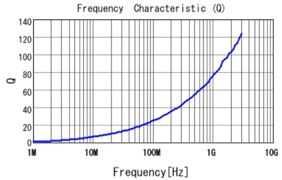
■ LQW15AN3N8G80 Q
