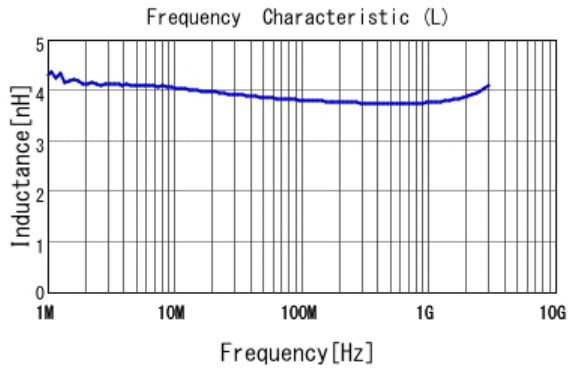
■ LQW15AN3N8G80 L
