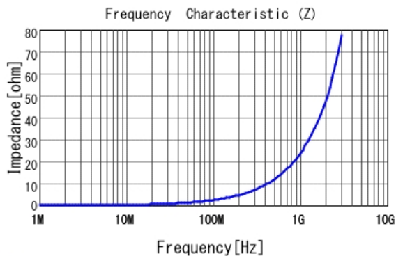
■ LQW15AN3N8G80 |Z|
