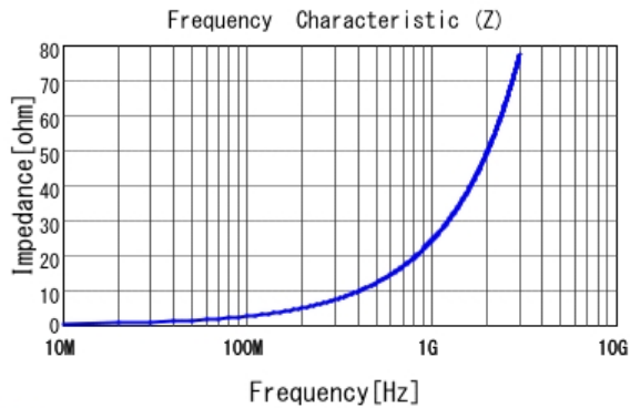
■ LQW15AN3N9B00 |Z|
