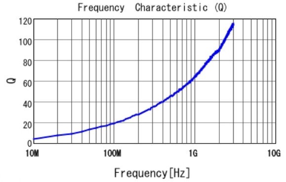
■ LQW15AN3N9B00 Q
