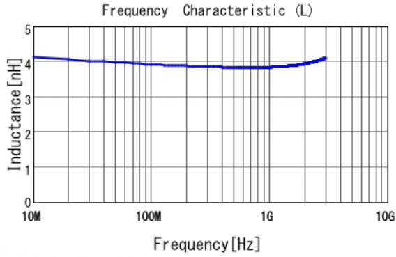
■ LQW15AN3N9B00 L
