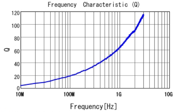
■ LQW15AN3N9C00 Q
