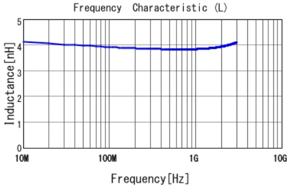
■ LQW15AN3N9C00 L
