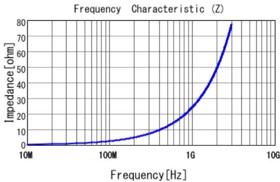
■ LQW15AN3N9C00 |Z|
