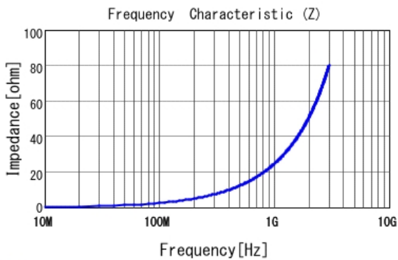
■ LQW15AN3N9D10 |Z|
