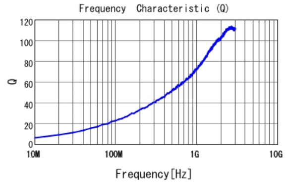
■ LQW15AN3N9D10 Q
