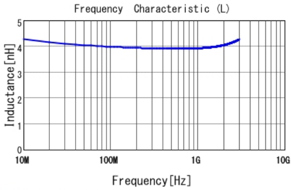
■ LQW15AN3N9D10 L
