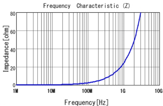
■ LQW15AN3N9G80 |Z|
