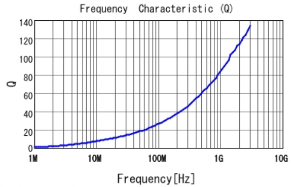
■ LQW15AN3N9G80 Q
