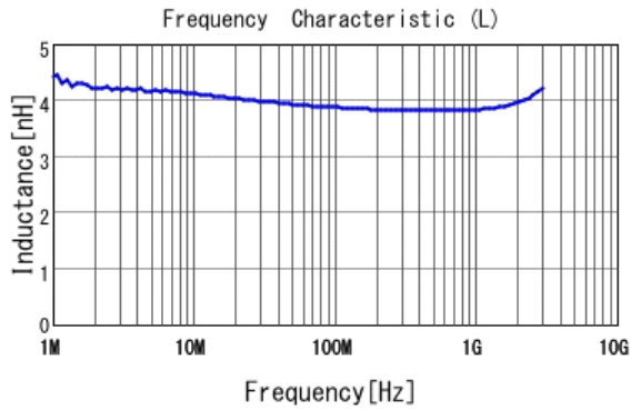
■ LQW15AN3N9G80 L
