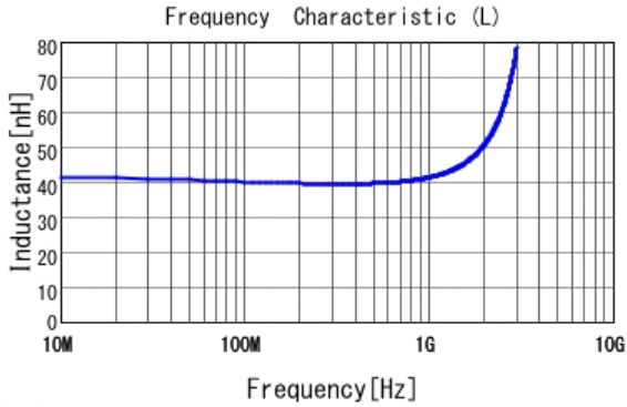
■ LQW15AN40NG00 L
