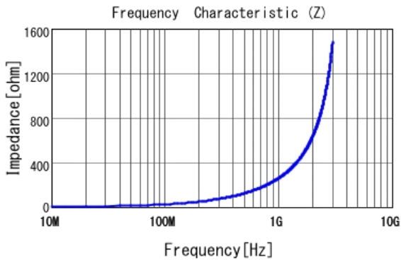
■ LQW15AN40NG00 |Z|
