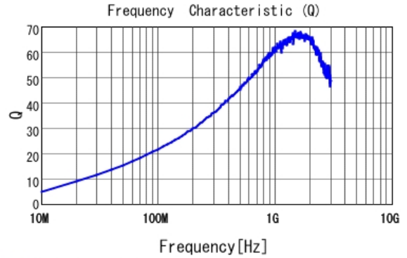
■ LQW15AN40NG00 Q
