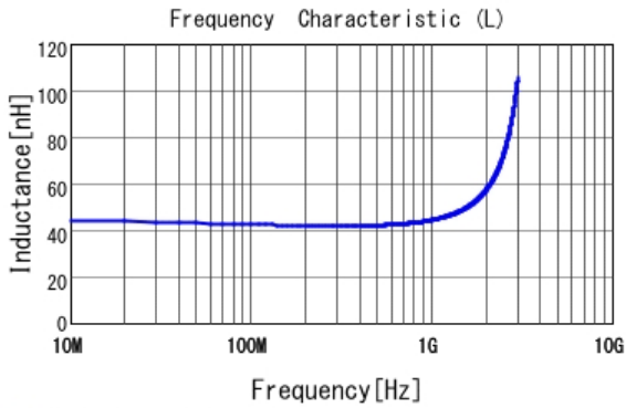
■ LQW15AN43NG00 L
