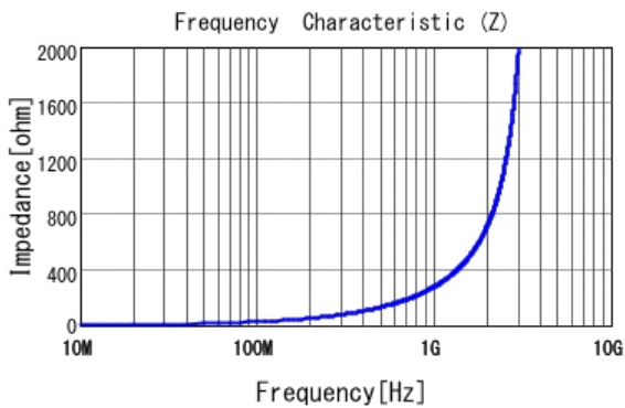
■ LQW15AN43NG00 |Z|
