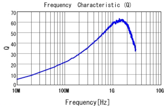
■ LQW15AN43NG00 Q
