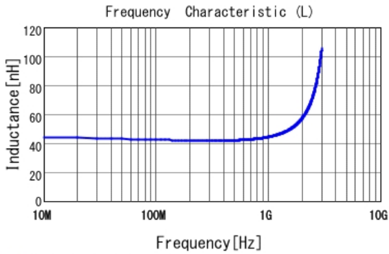
■ LQW15AN43NJ00 L
