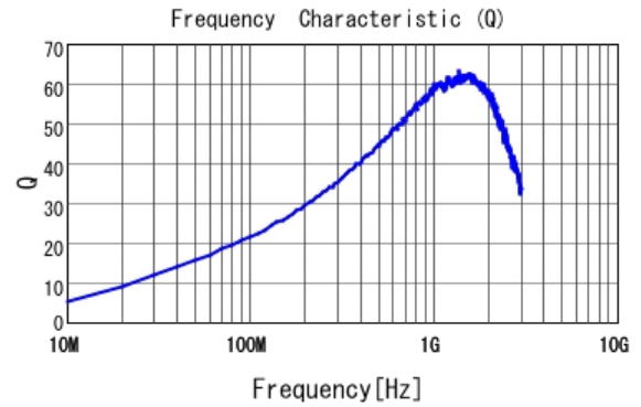
■ LQW15AN43NJ0Z Q
