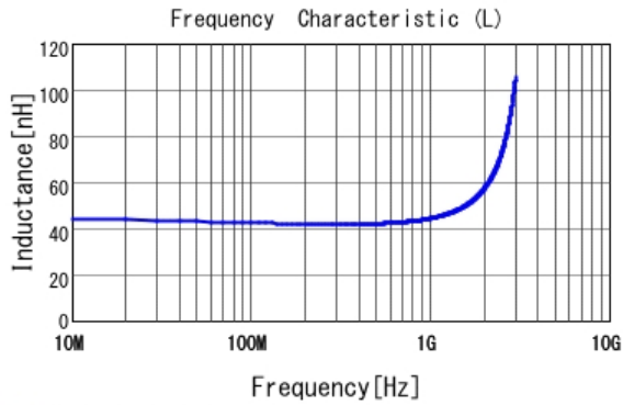
■ LQW15AN43NJ0Z L
