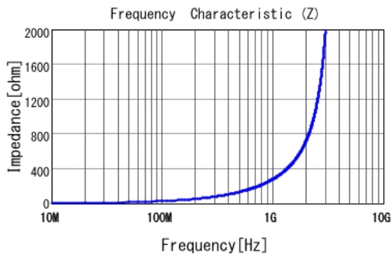
■ LQW15AN43NJ0Z |Z|
