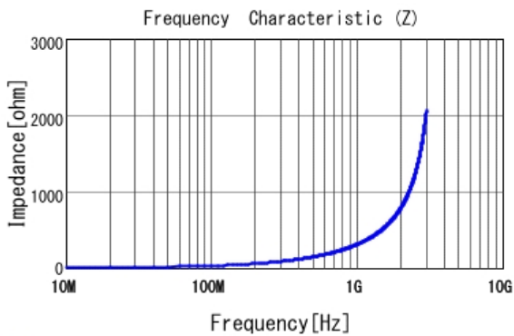
■ LQW15AN47NG00 |Z|
