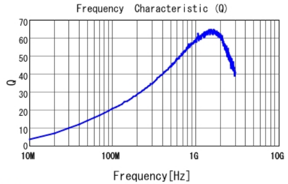
■ LQW15AN47NG00 Q
