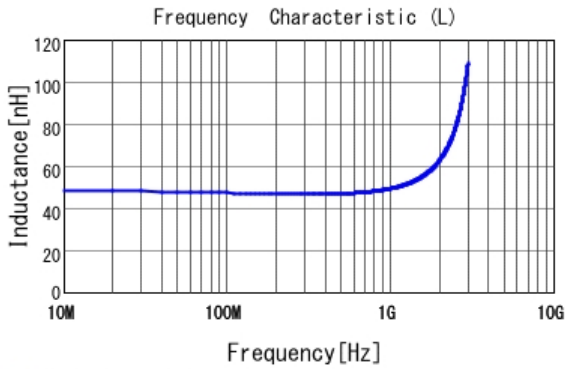
■ LQW15AN47NG00 L
