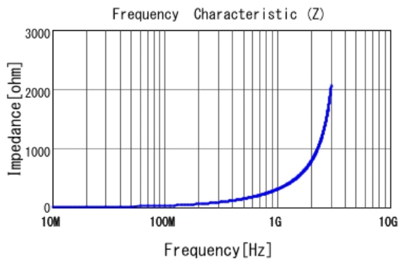
■ LQW15AN47NJ00 |Z|
