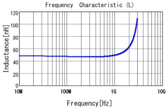
■ LQW15AN47NJ00 L
