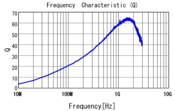
■ LQW15AN47NJ00 Q
