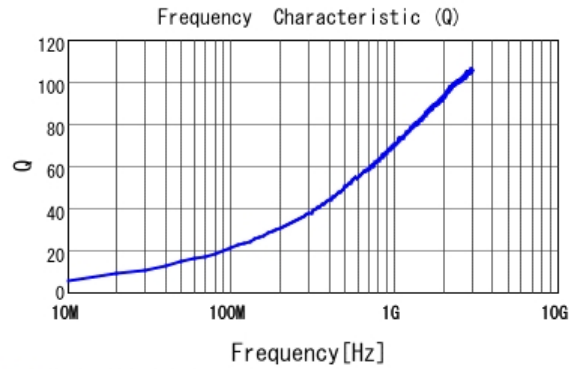
■ LQW15AN4N0C10 Q
