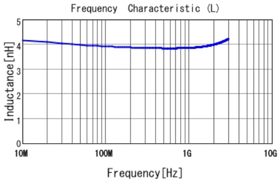
■ LQW15AN4N0C10 L
