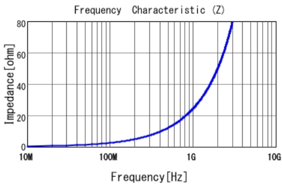
■ LQW15AN4N0C10 |Z|
