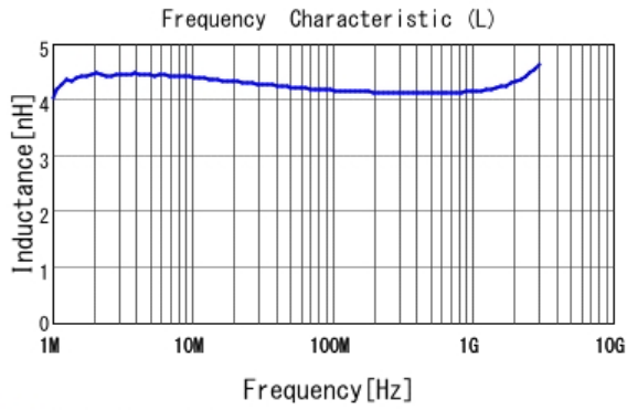
■ LQW15AN4N1G80 L
