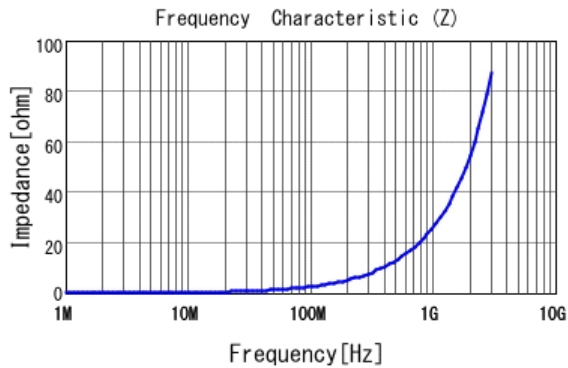
■ LQW15AN4N1G80 |Z|
