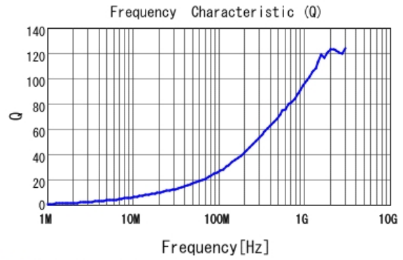
■ LQW15AN4N1G80 Q
