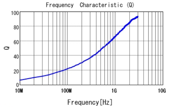
■ LQW15AN4N2C10 Q
