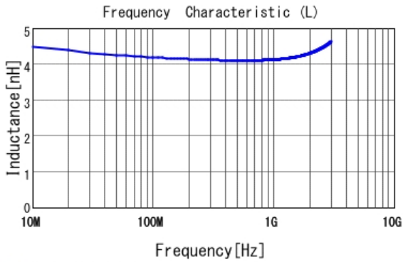
■ LQW15AN4N2C10 L
