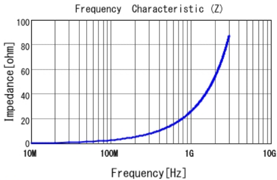
■ LQW15AN4N2C10 |Z|
